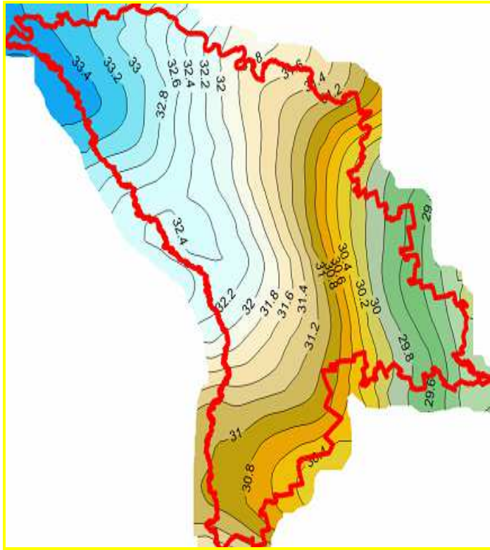
Fig.3. Modelul suprafeței de referință al altitudinilor HRS.
